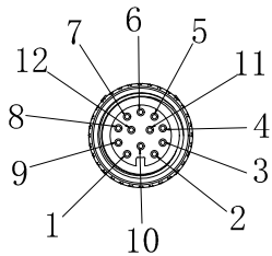
M12防水航空插头线序
