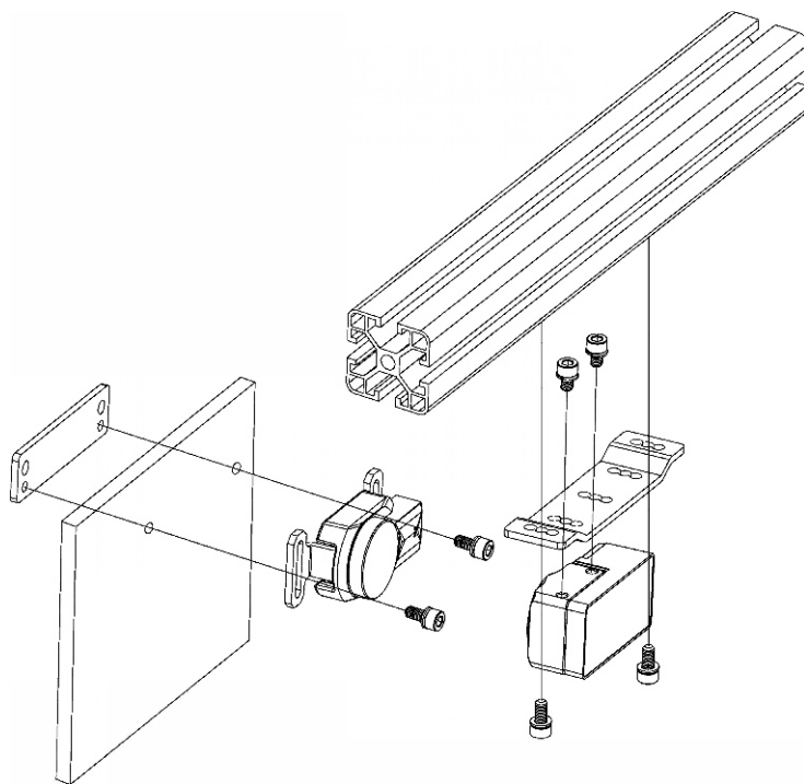
匹配器可动面板安装
