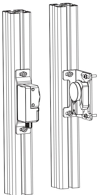
匹配器可动框架安装
